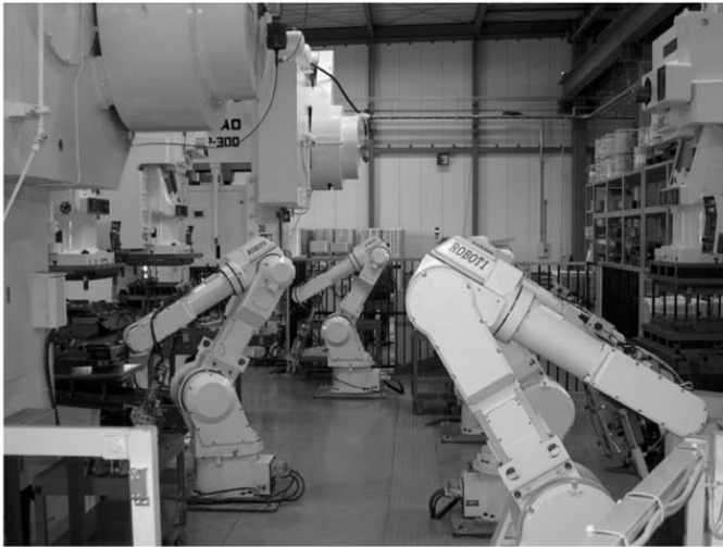
多軸ロボット6台ライン ▲
